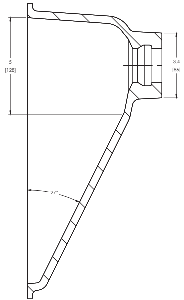
SECTION B-B SCALE: FULL
