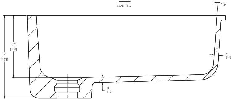
SECTION A-A SCALE: FULL
